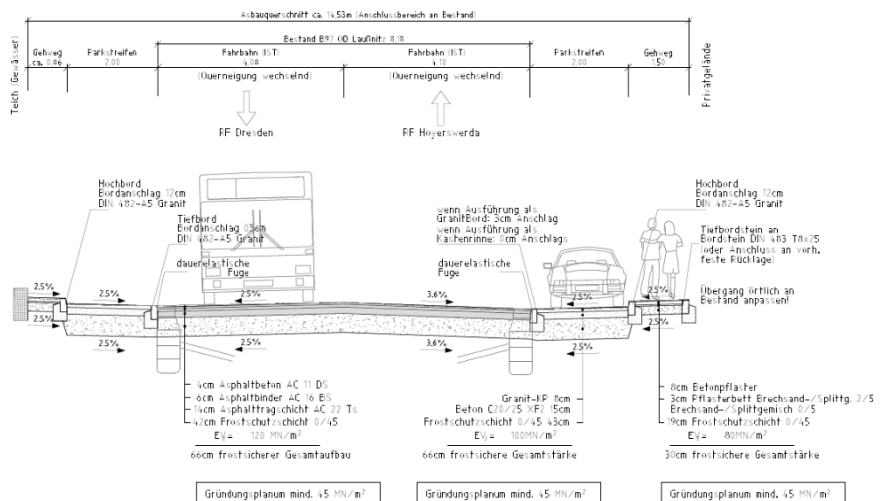
RQ: Ausbauquerschnitt der B 97(Bereich mit angrenz. Bebauung)
