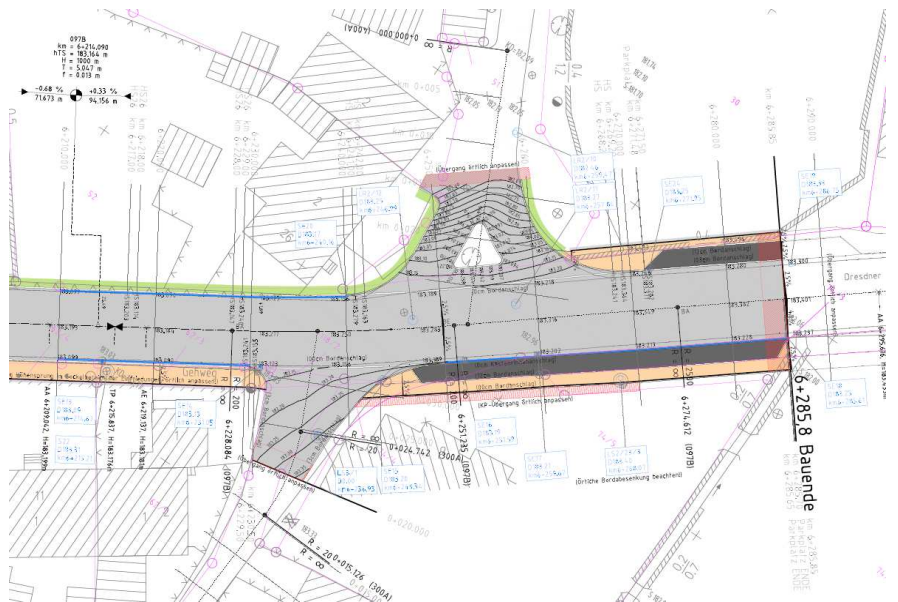
LP: Ausbaubereich mit Gradientenabsenkung und Einmündungen
