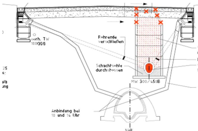
Schnitt Uferstraße mit Neustädter Abfangkanal
