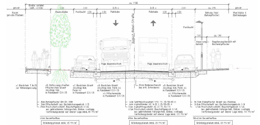
Querungsstelle 1 M 1:50
