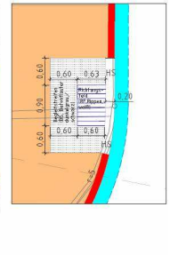
Querungsstelle 3 M 1:50
