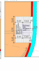
Querungsstelle 3 M 1:50
