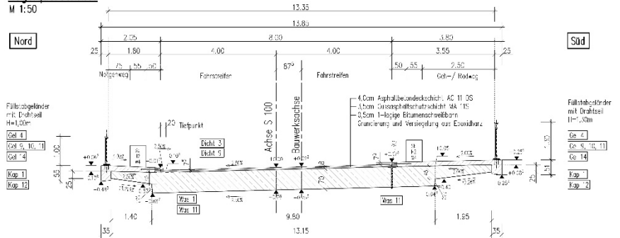
Regelquerschnitt
