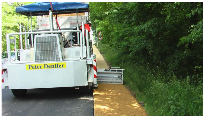
Banketteinbau mit Fertiger
